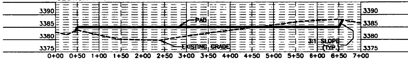
SECTION A-A'
