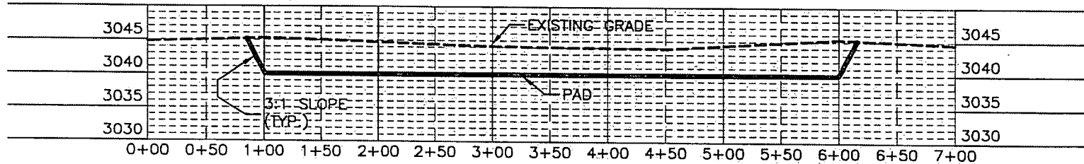
SECTION A-A'
