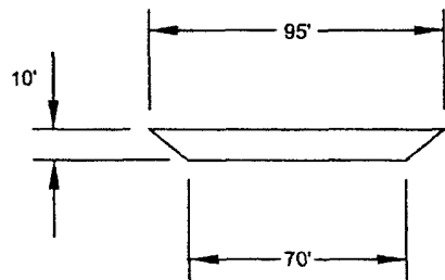
VIEW A-A
