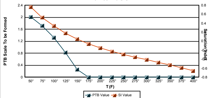
Celestite \text{SrSO}_4
