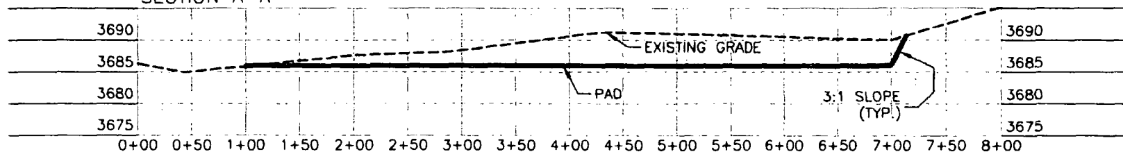
SECTION A-A'
