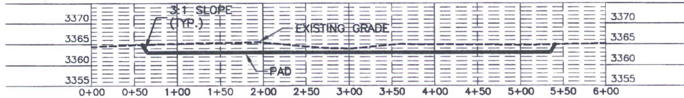
SECTION A-A'
