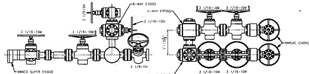
VIEW A-A
