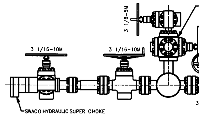
VIEW A-A
