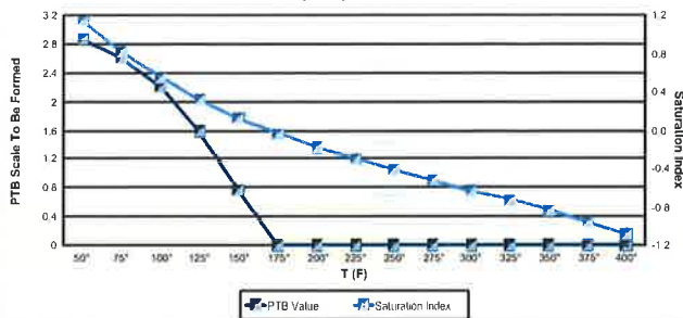
Celestite SrSO4
