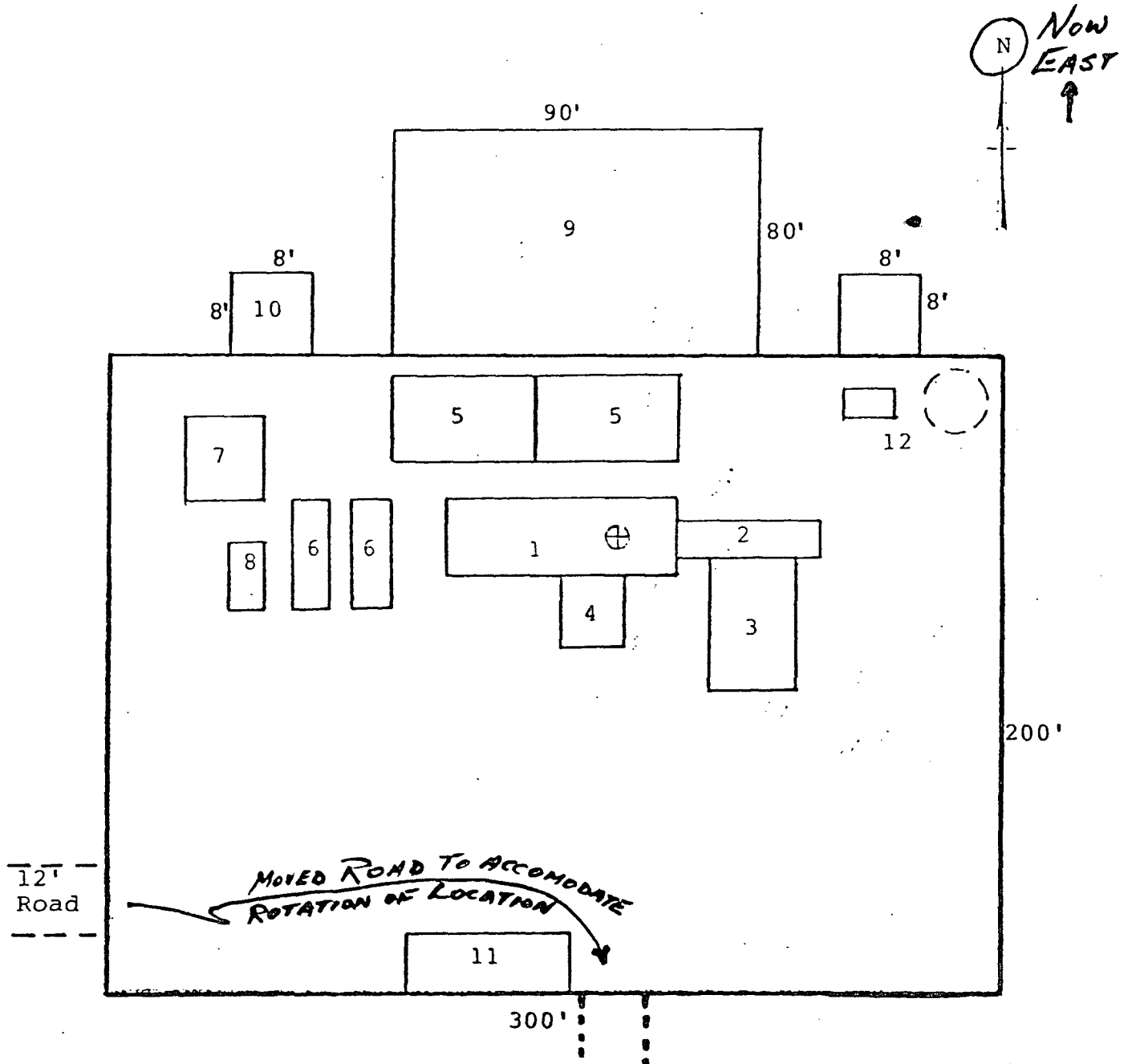
RIG LAYOUT
