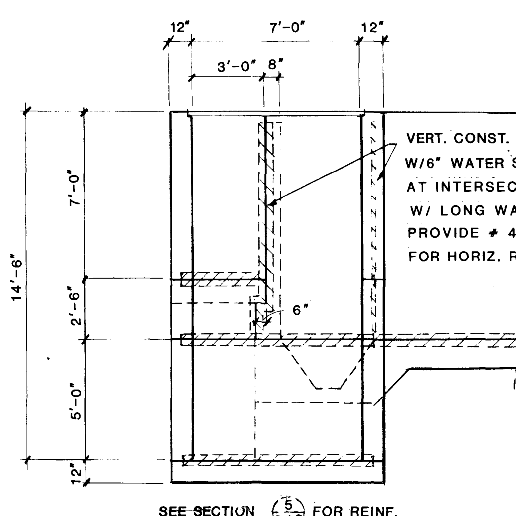
SECTION 6 SCALE: 1/4" 1'-0"
