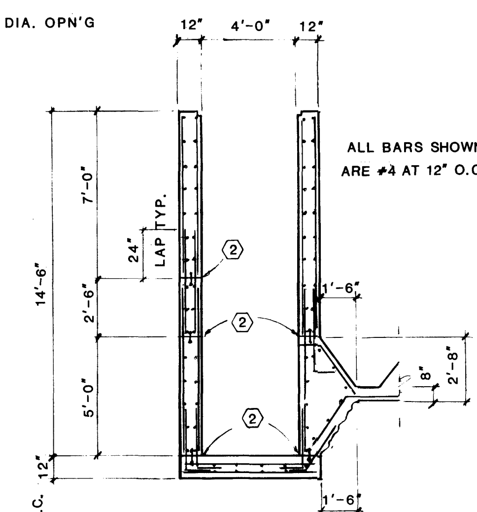
SECTION 5 SCALE: 1/4" 1'-0"
