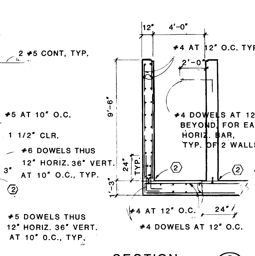
SECTION 3 SCALE: 1/4" 1'-0"
