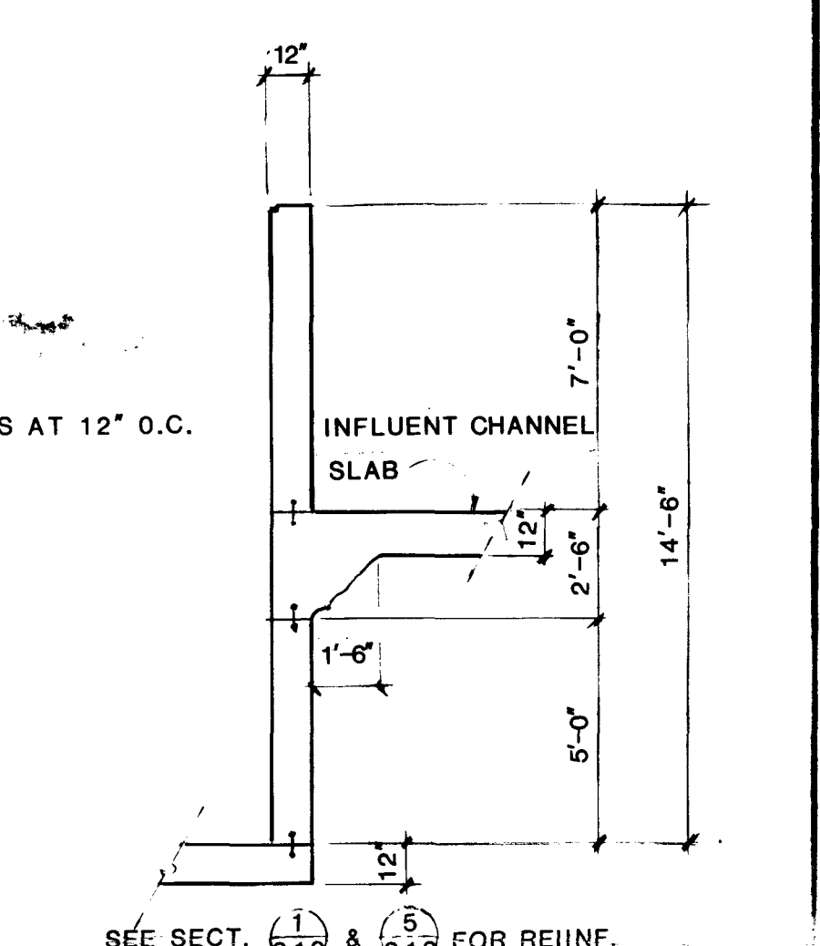
SECTION 7 SCALE: 1/4" 1'-0"
