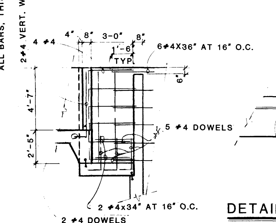
SECTION 8 SCALE: 1/4" 1'-0"
