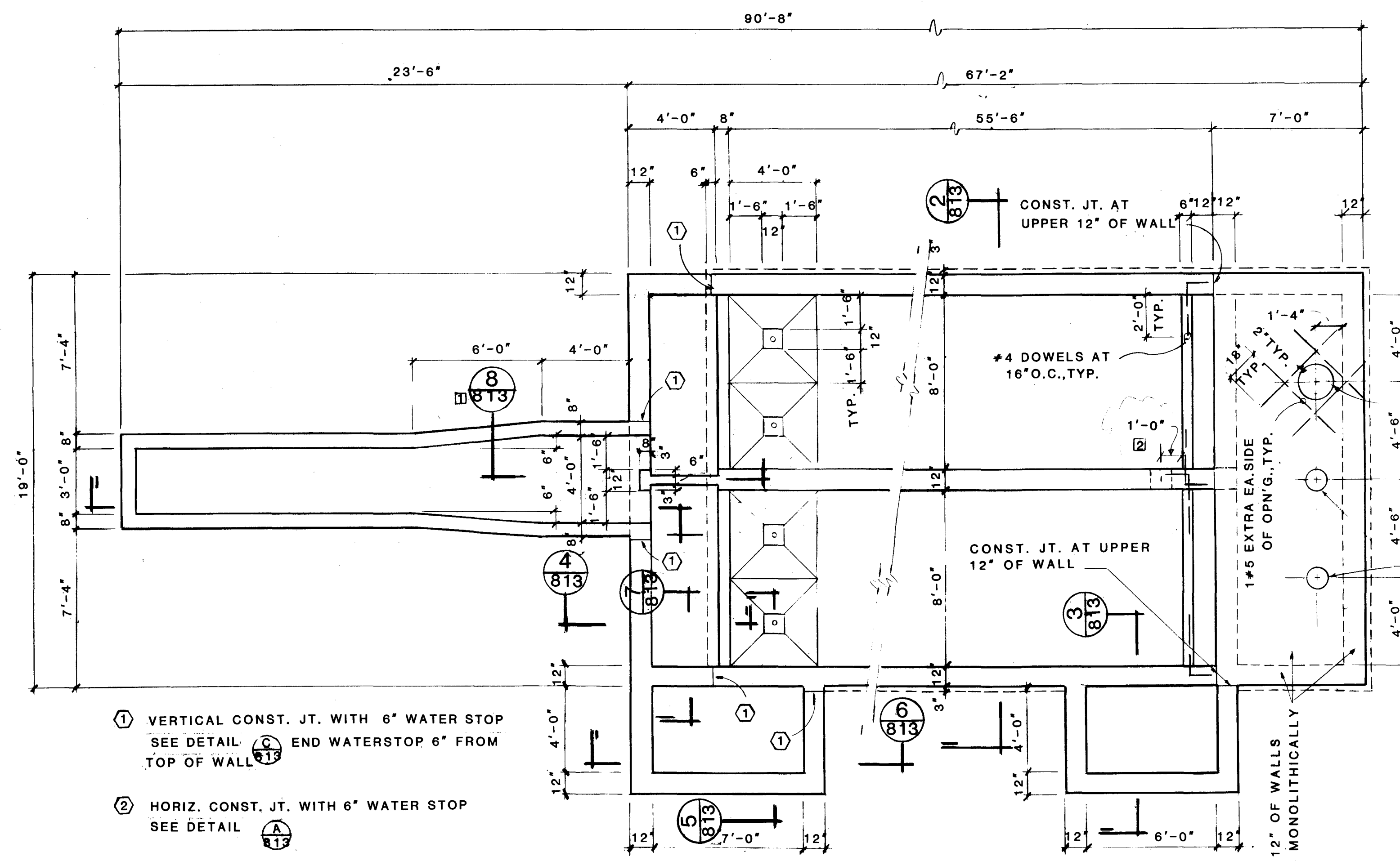
PLAN SCALE: 1/4" 1'-0"
