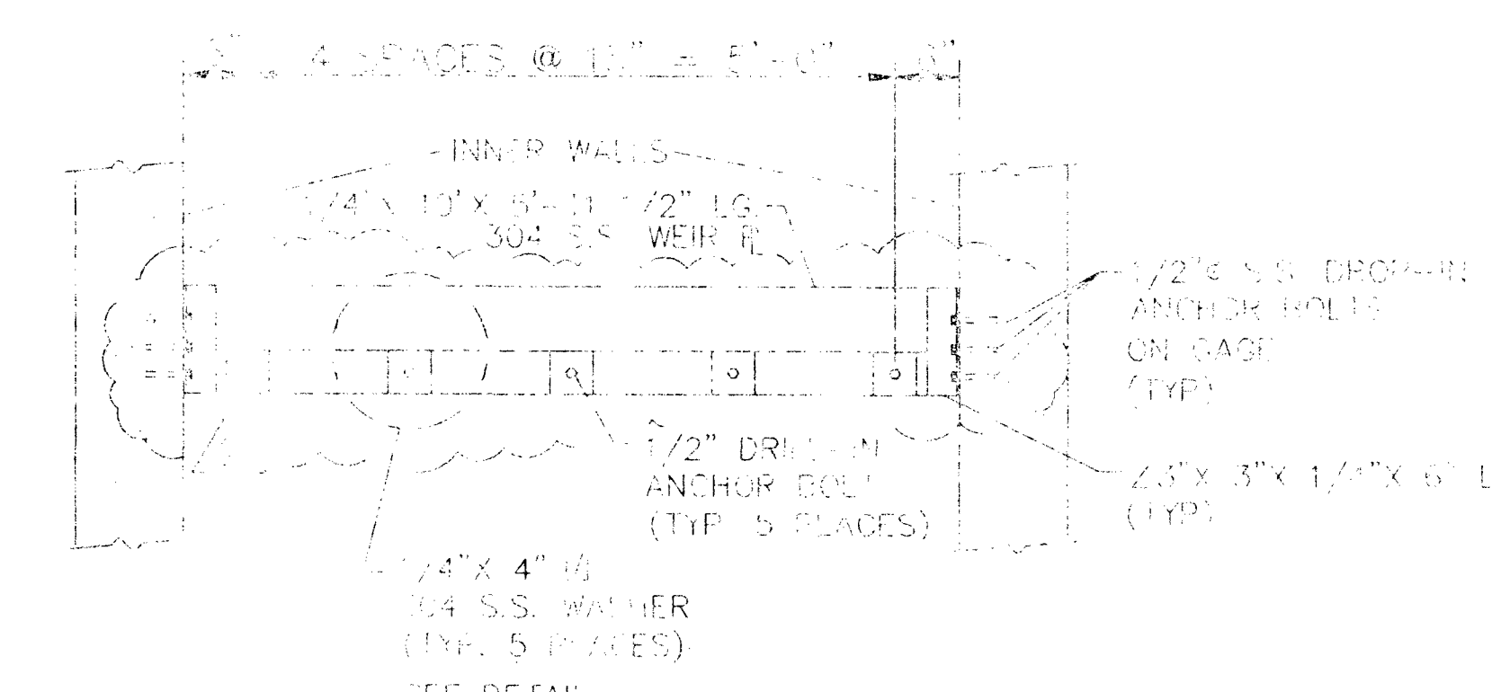
ELEVATION SCALE: 3/4" = 1'-0"
