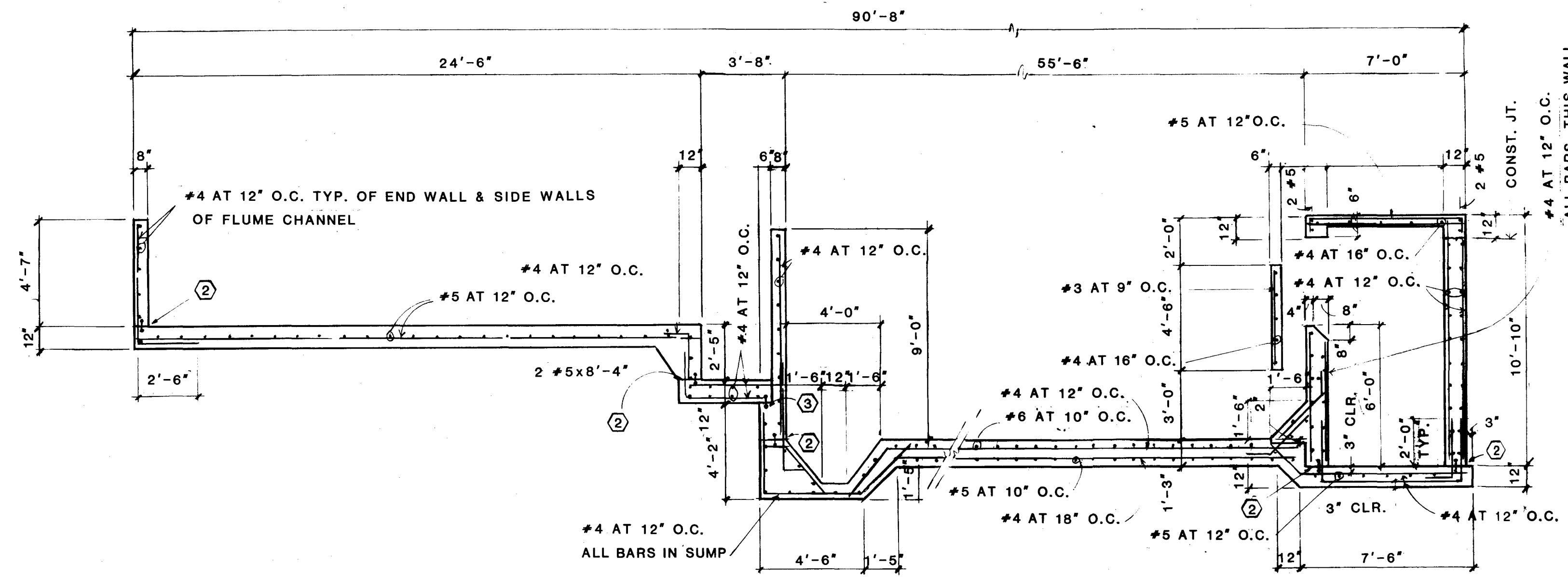
SECTION 1 SCALE: 1/4" 1'-0"
