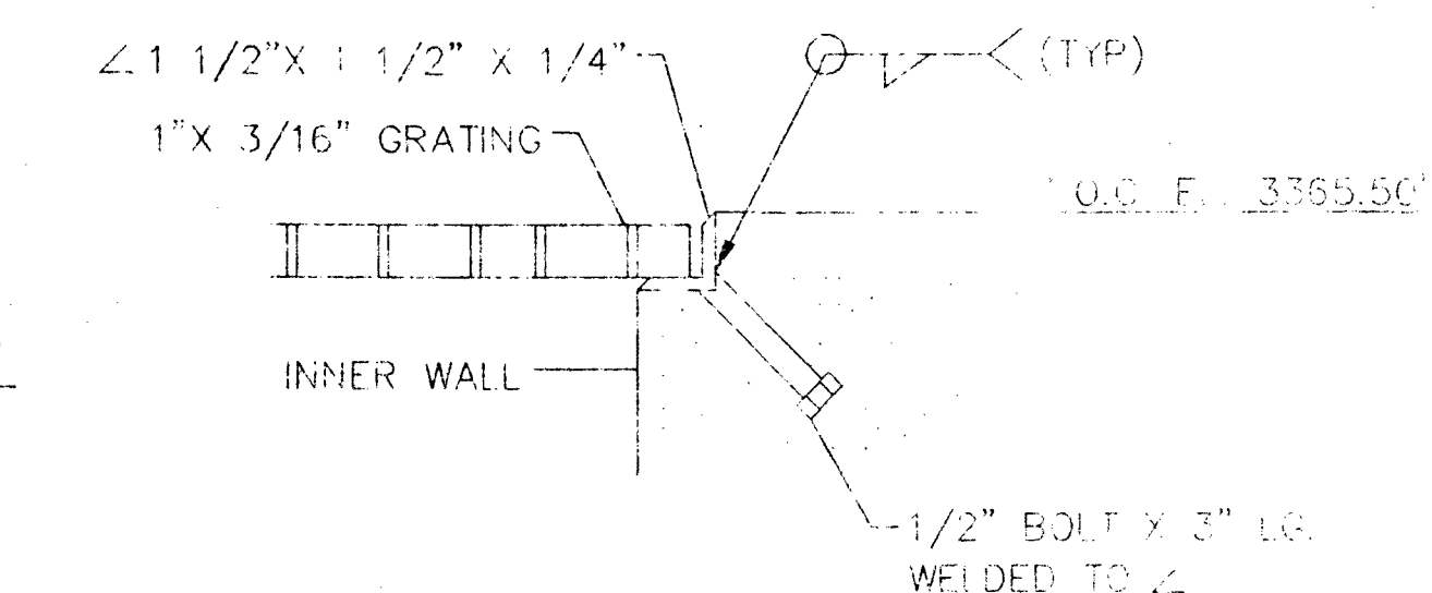
DETAIL "2" SCALE: 3" = 1'-0"
