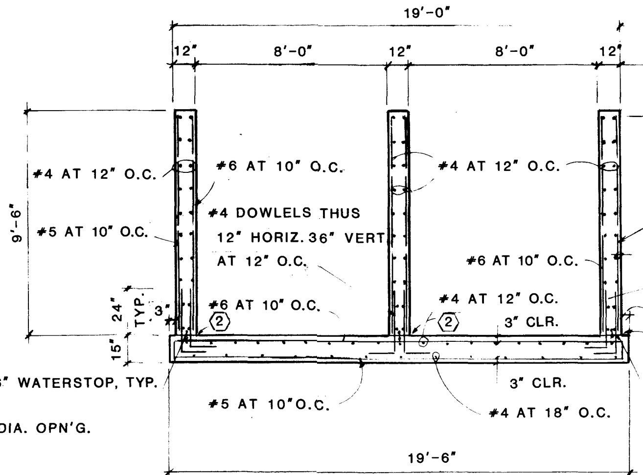
SECTION 2 SCALE: 1/4" 1'-0"
