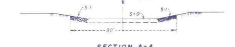
SECTION A-A
