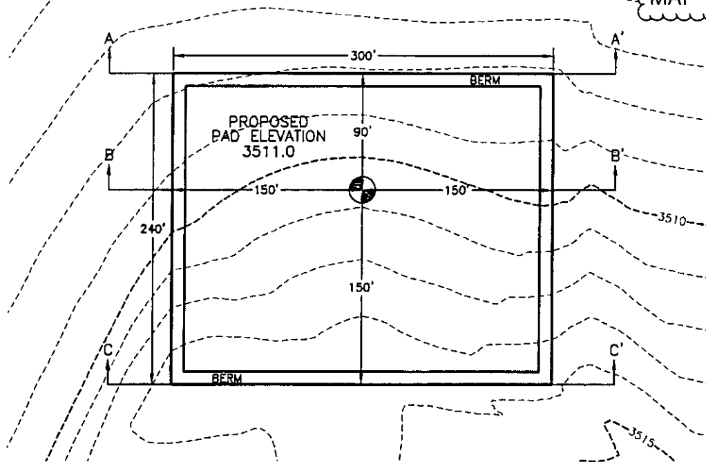
SECTION A-A'
