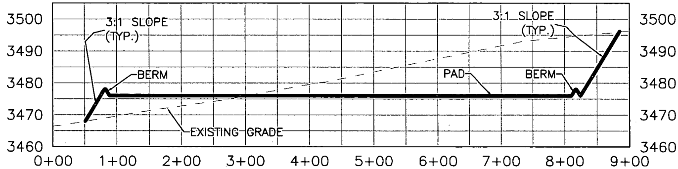
SECTION D-D
