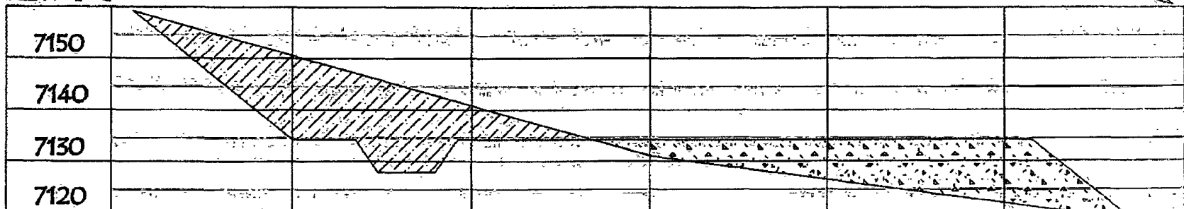
ELEV. C'-C
