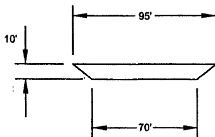
VIEW A-A
