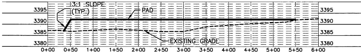
SECTION A-A'
