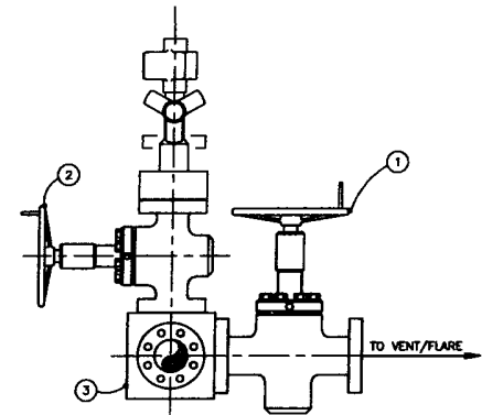
VIEW A-A
