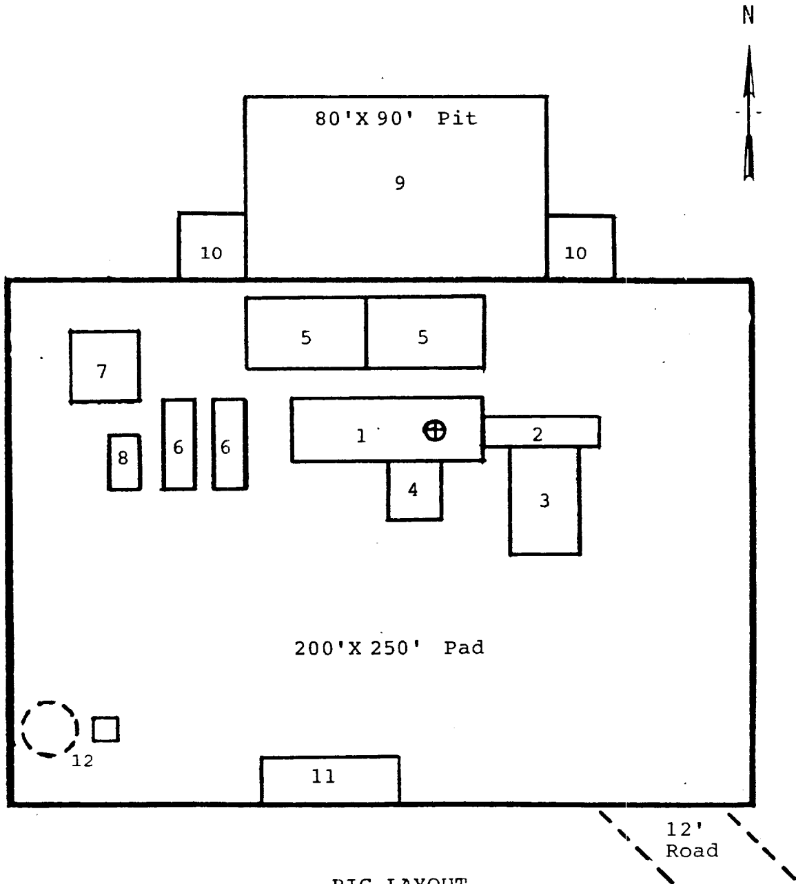
RIG LAYOUT
