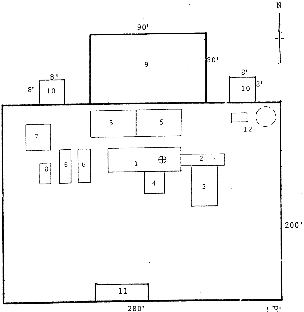
RIG LAYOUT
