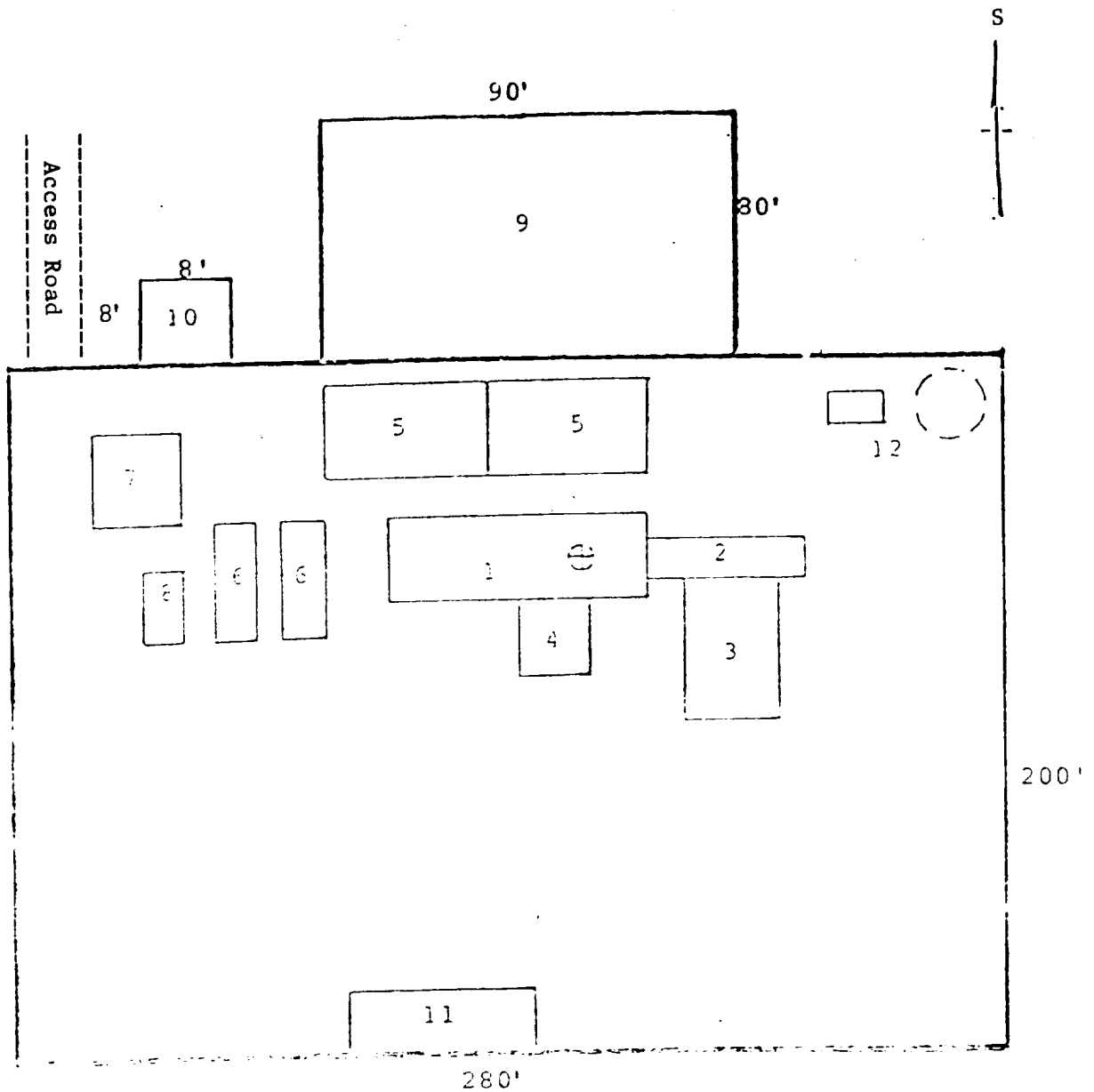
RIG LAYOUT
