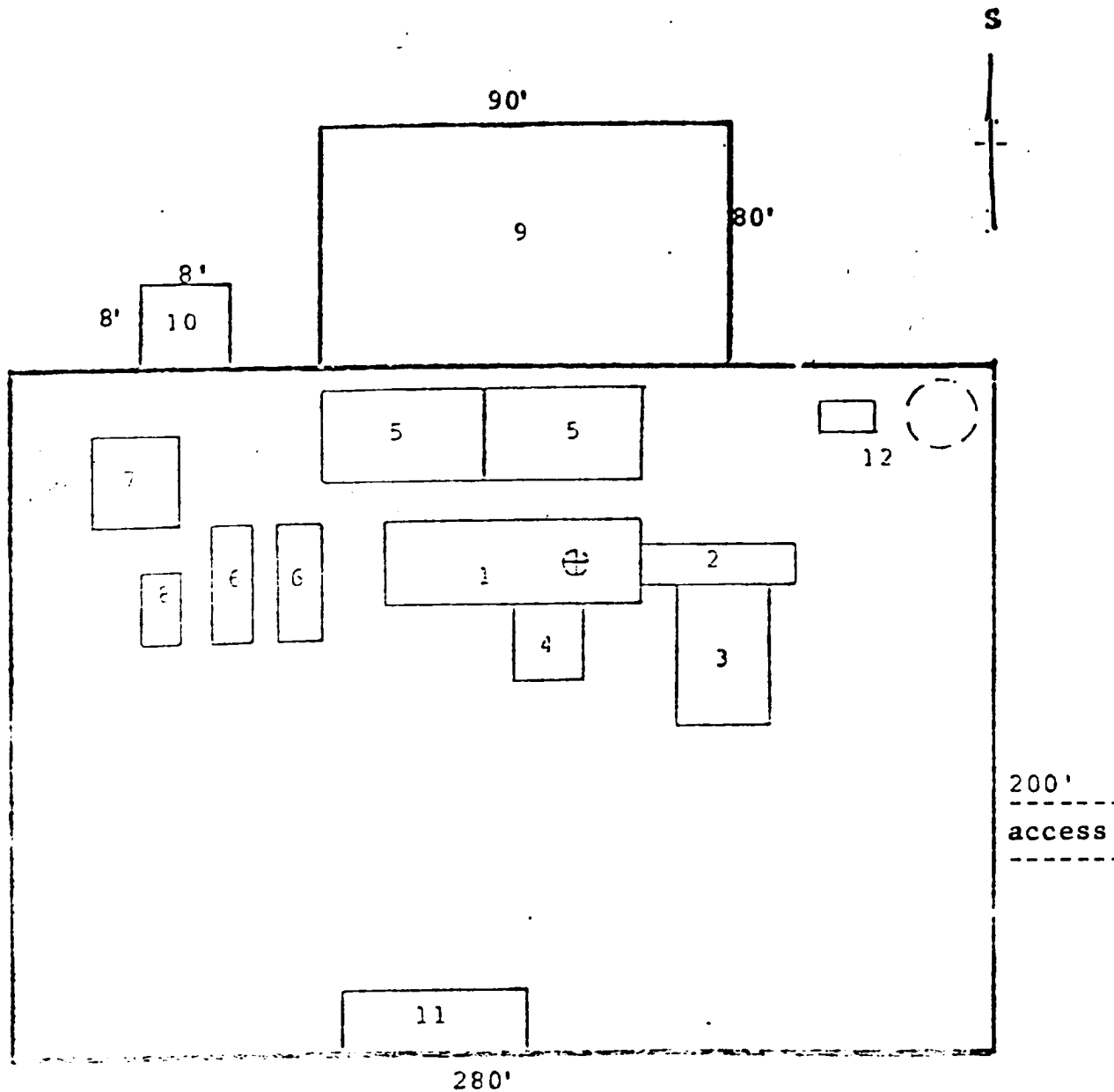
RIG LAYOUT
