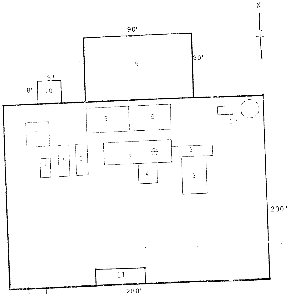
RIG LAYOUT
