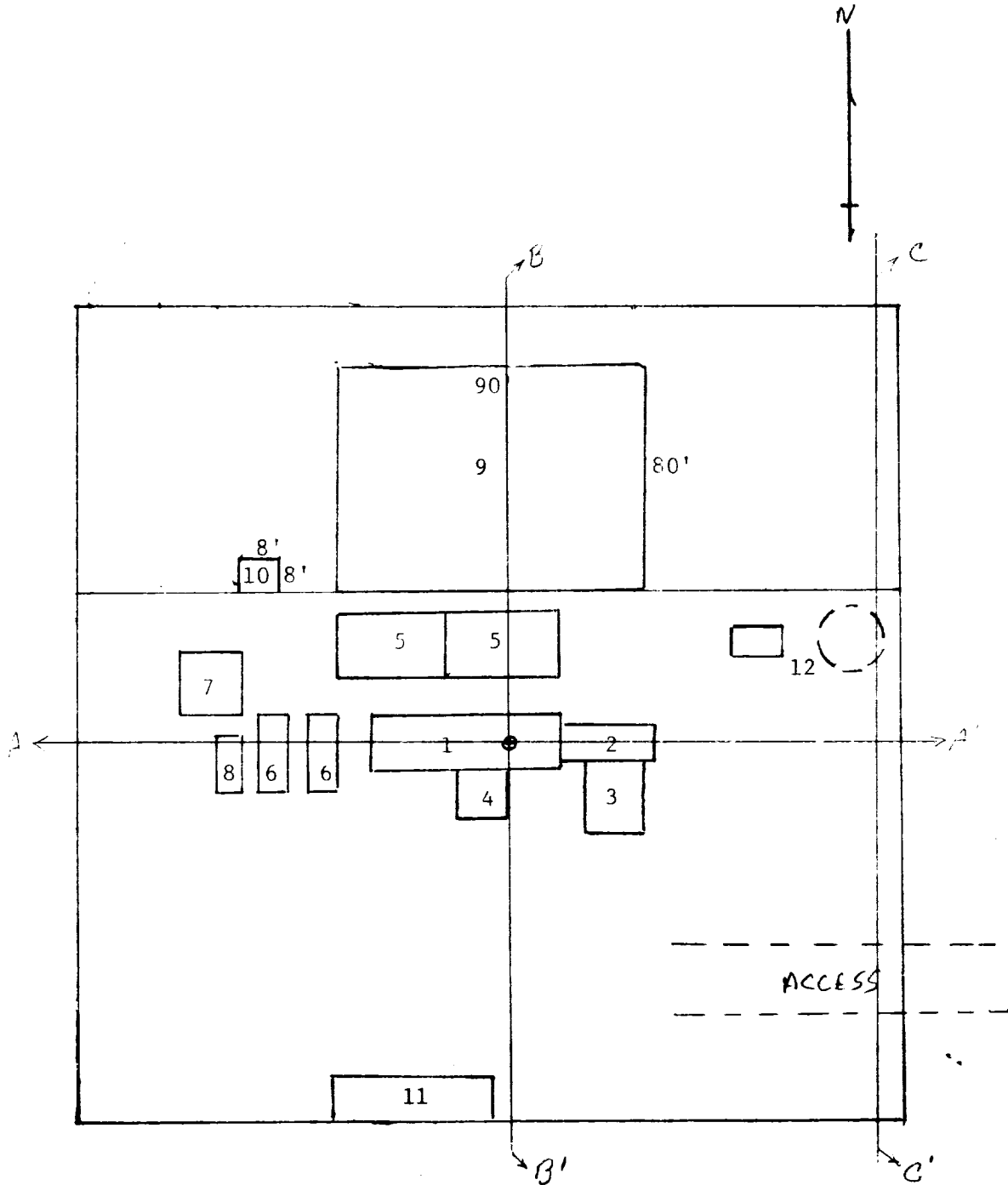
RIG LAYOUT
