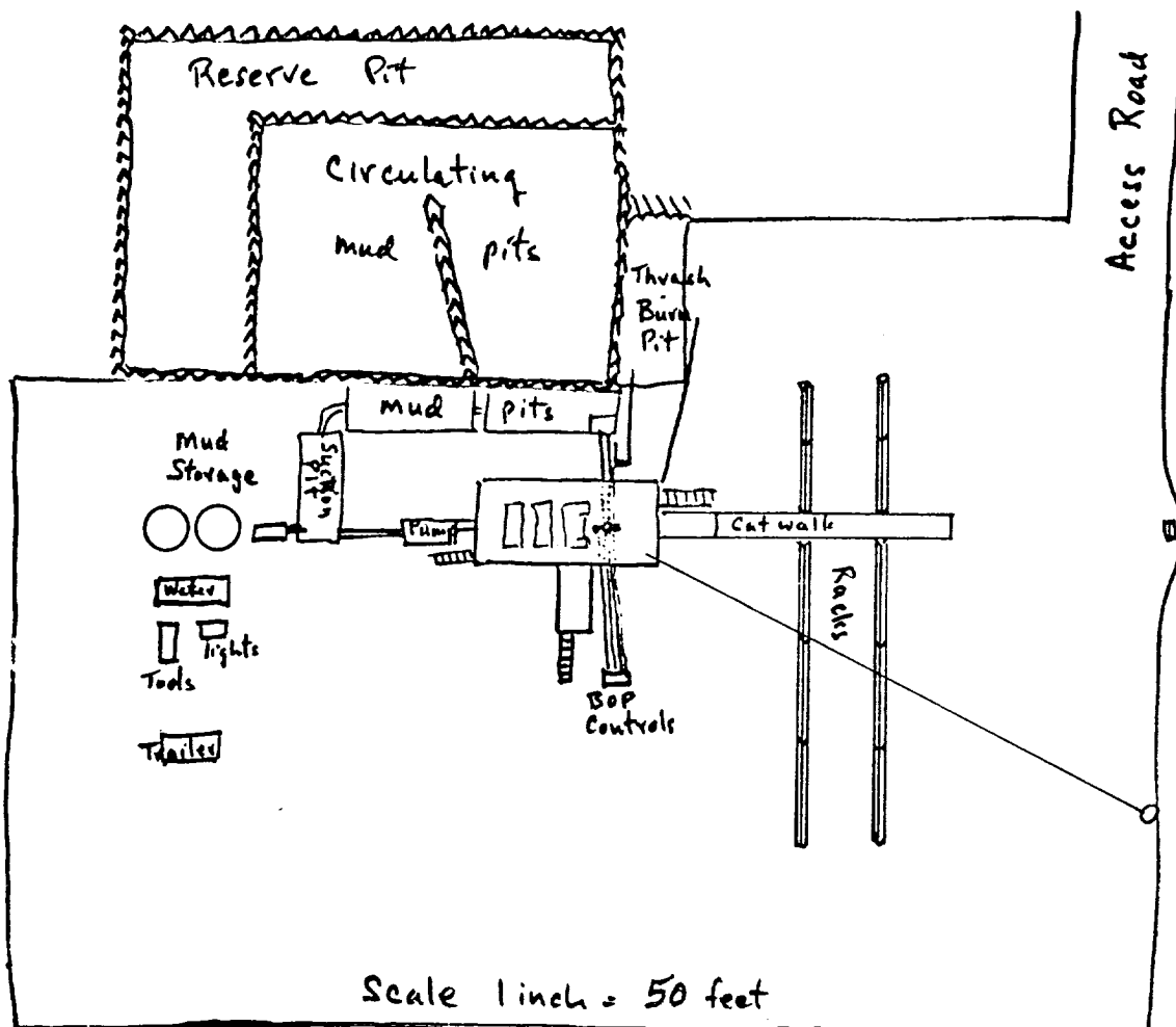
Rig Layout
