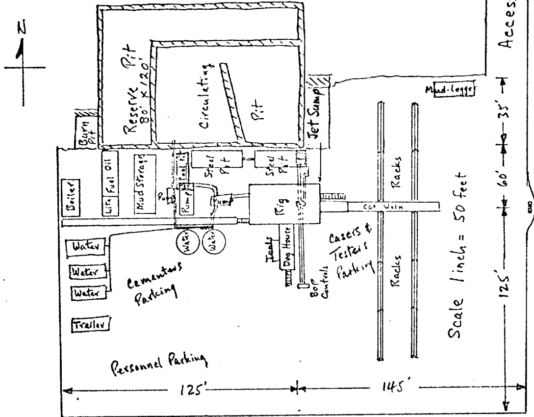
Rig layout
