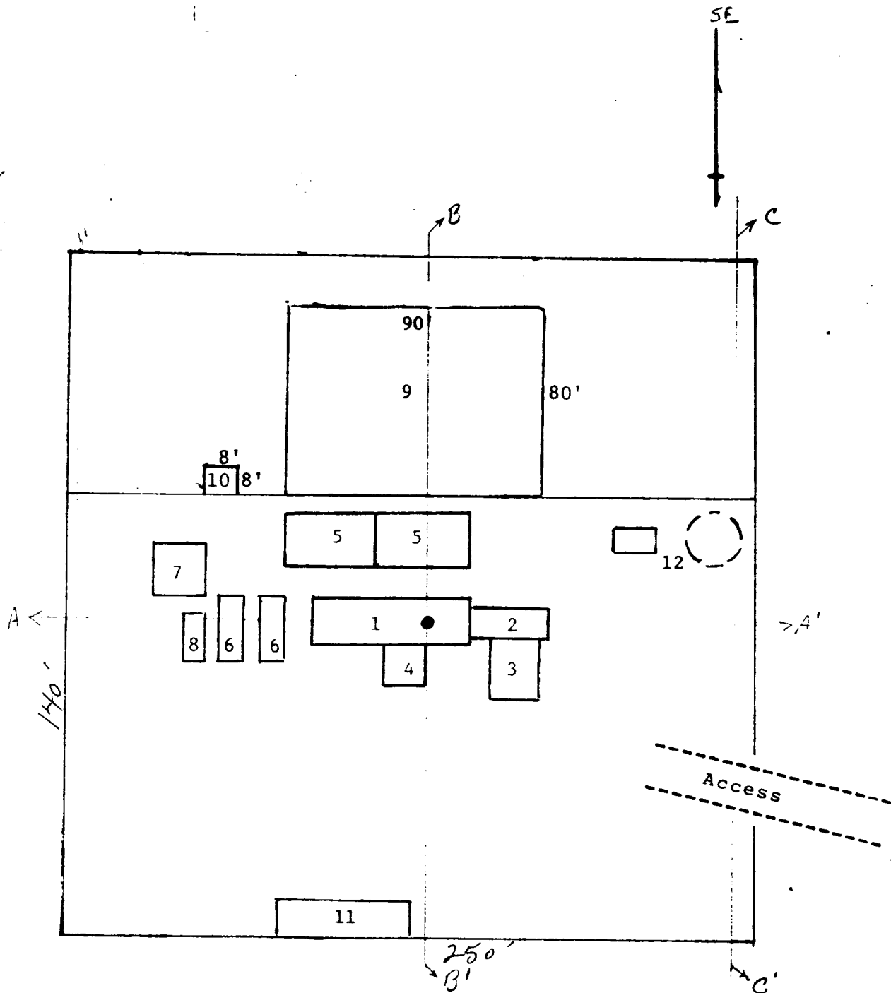
RIG LAYOUT
