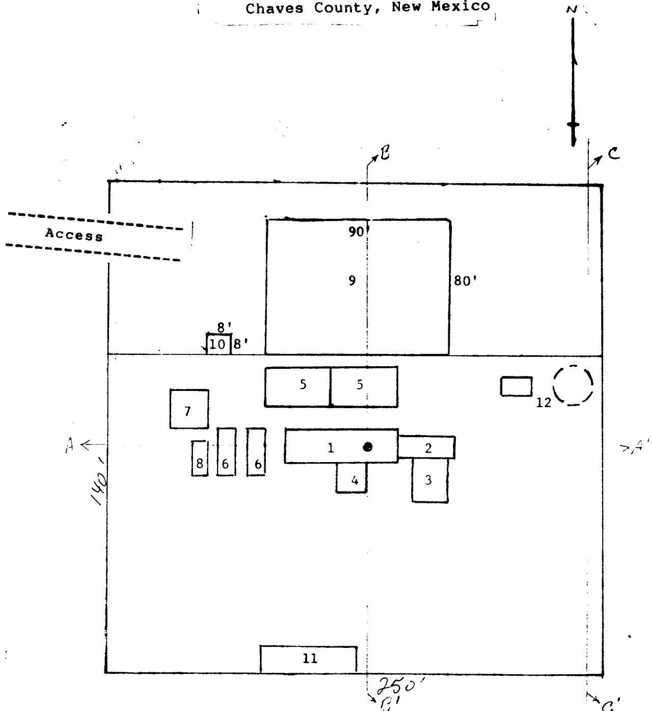
RIG LAYOUT
