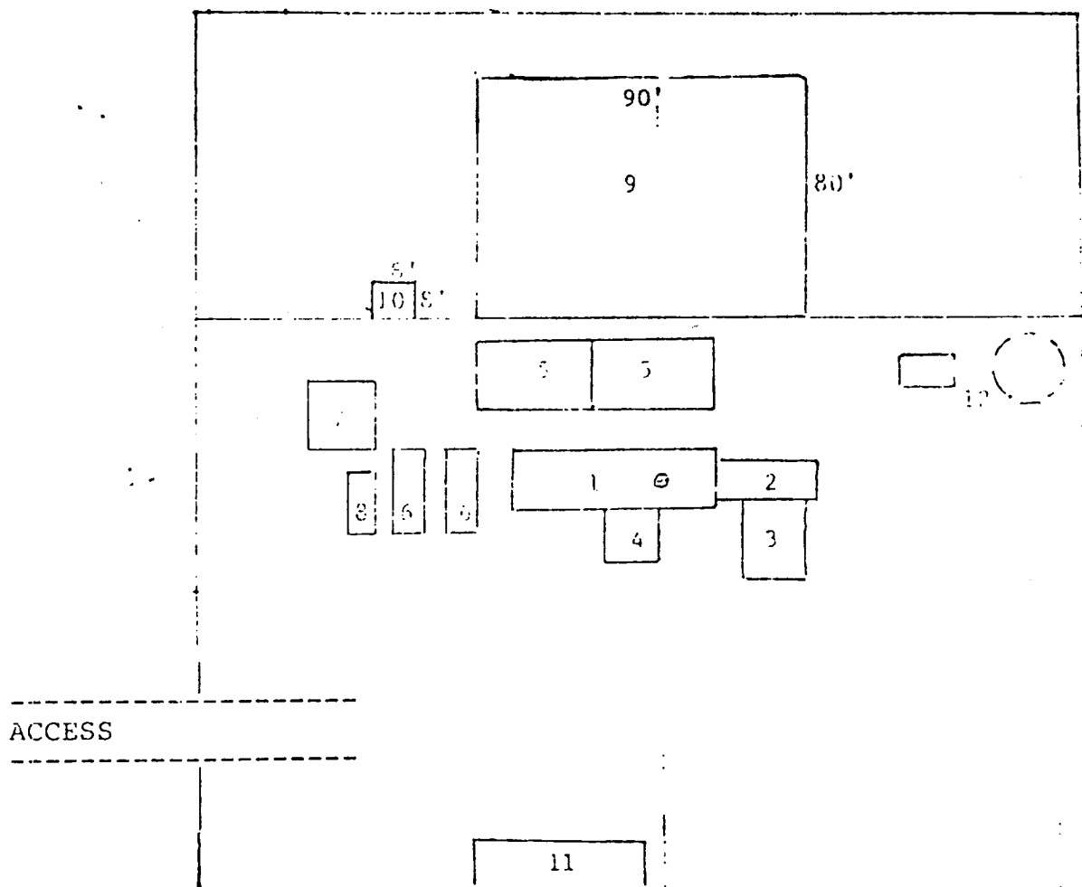
RIG LAYOUT
