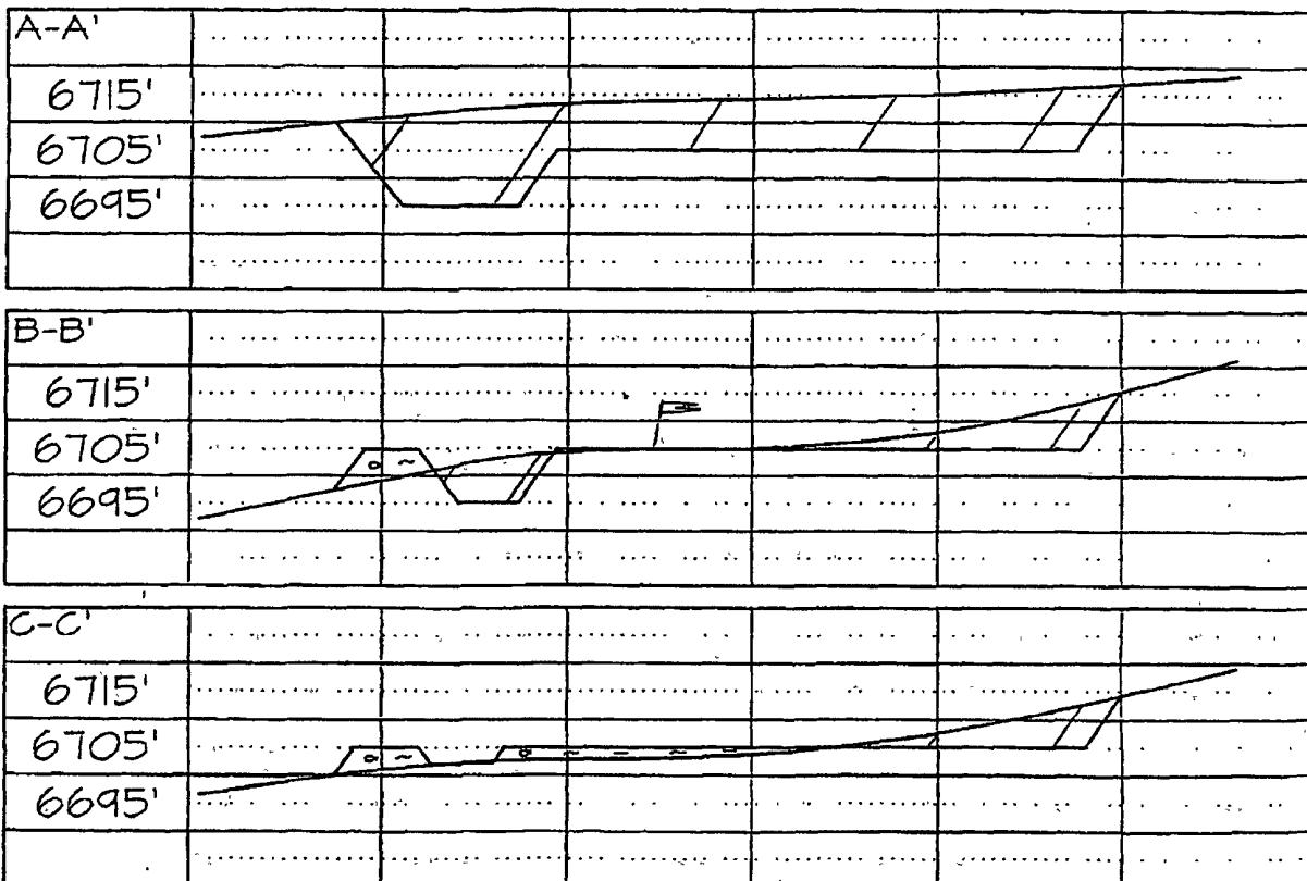
Plat #2 cut/fill
