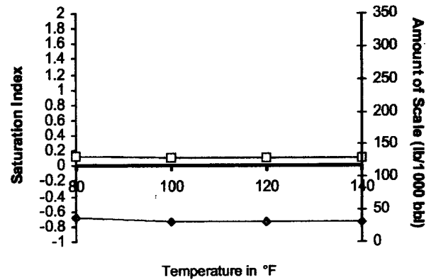
Celestite - \text{SrSO}_4
