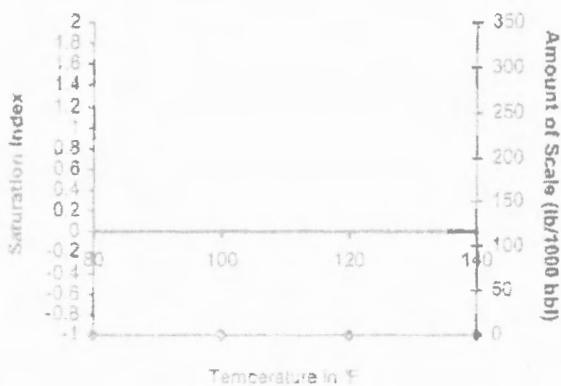
Celestite - \text{SrSO}_4
