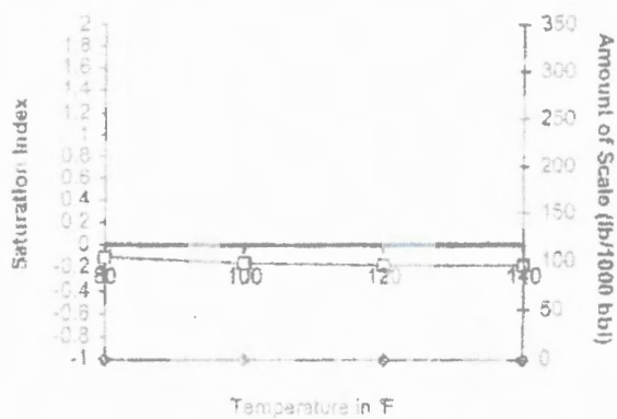
Celestite - \text{SrSO}_4
