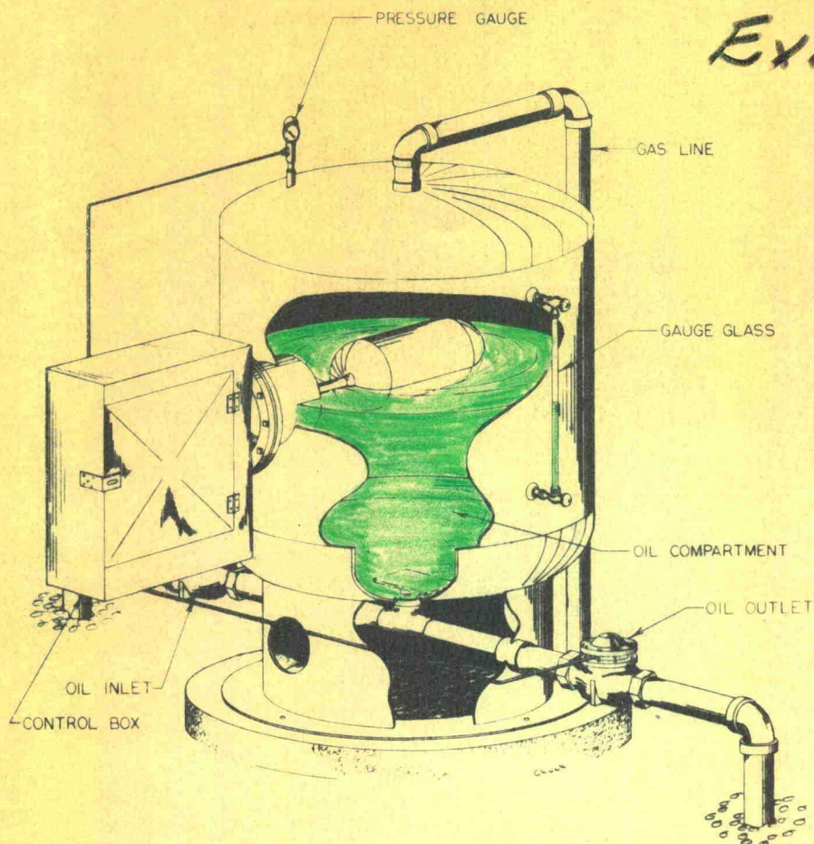
SIVALLS DUMP METER
