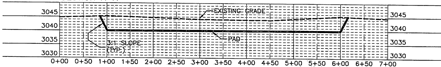
SECTION A-A'
