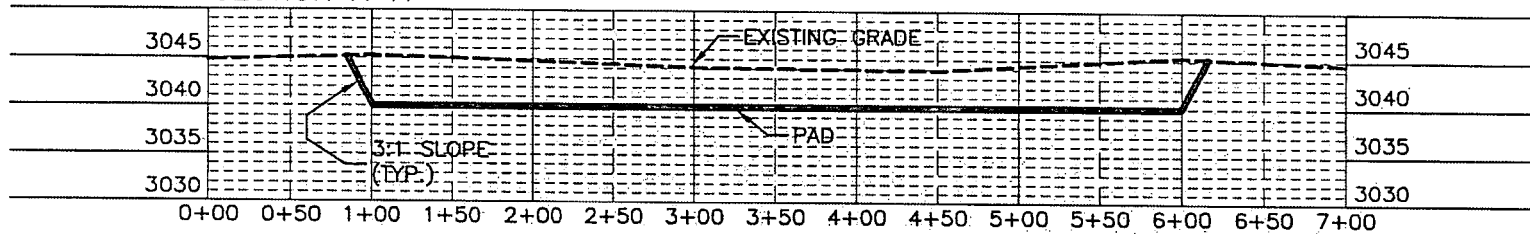
SECTION A-A'
