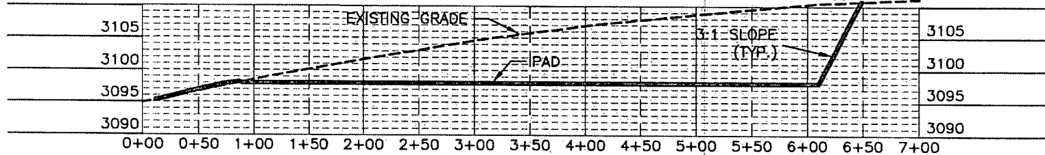
SECTION A-A'
