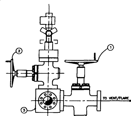
VIEW A-A
