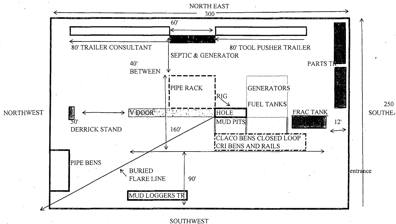
Gissler B 68 Rig Layout
