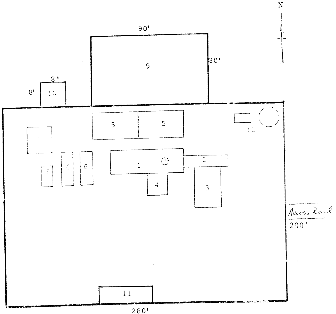
RIG LAYOUT
