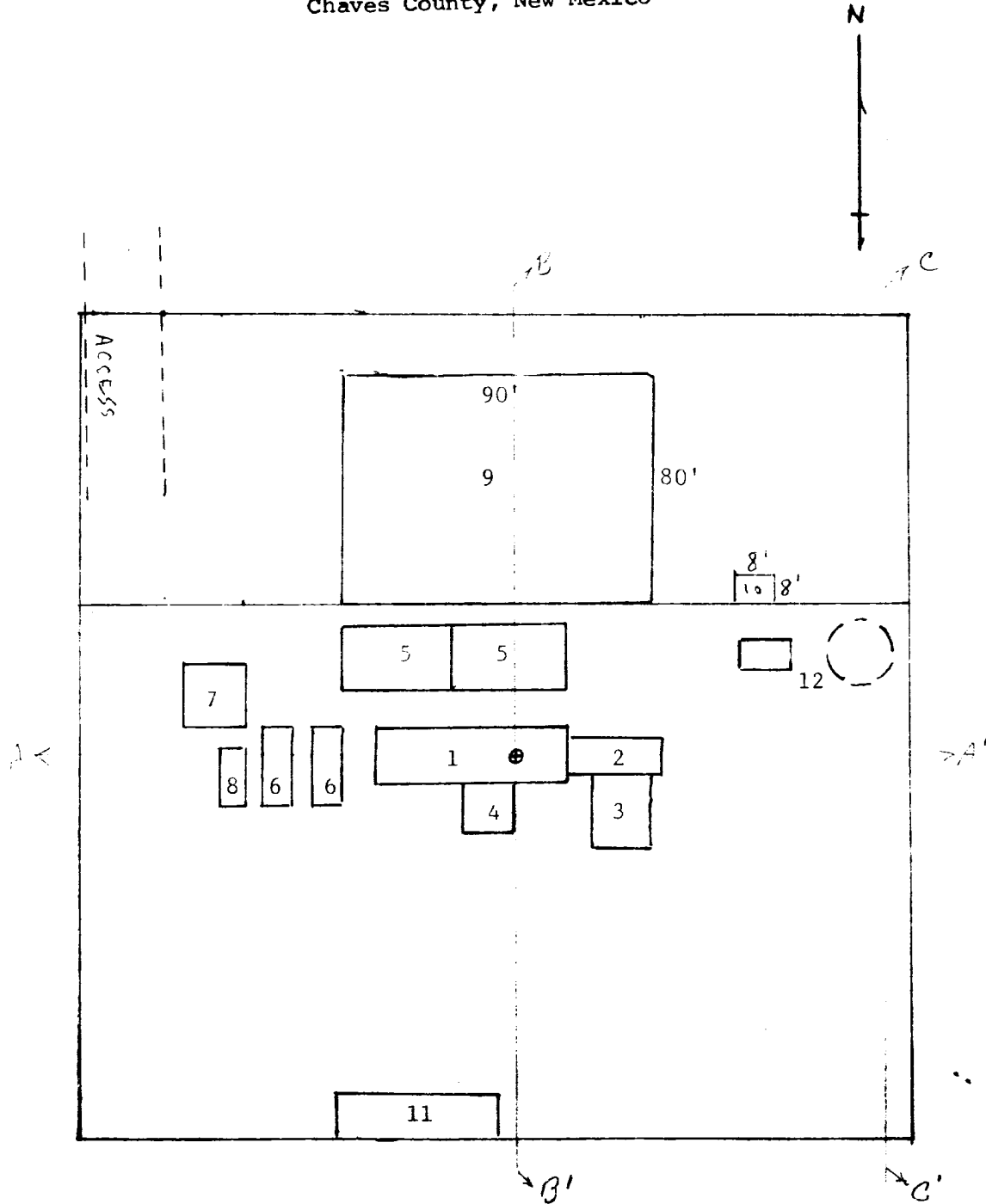
RIG LAYOUT
