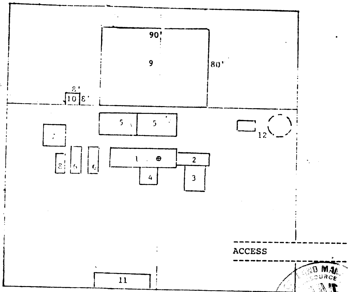
RIG LAYOUT
