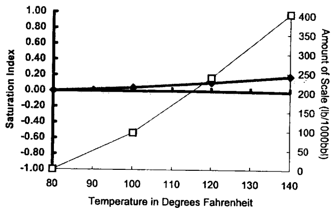
Anhydrite - \text{CaSO}_4
