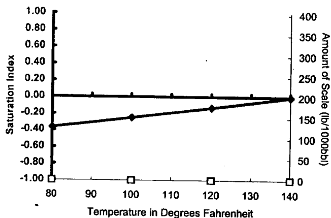
Calcite - \text{CaCO}_3
