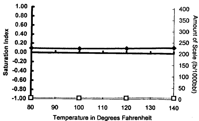
Celestite - \text{SrSO}_4
